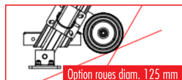
Platines articulées en tôle larmée de 5,5 mm
